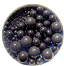
Si 3 N 4
