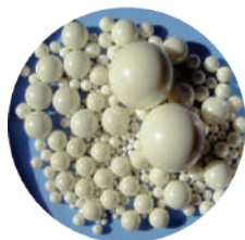
ZrO 2
